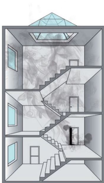
Rys. 1. Budynek bez okiennego systemu oddymiania mcr OSO
