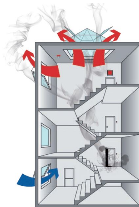
Rys. 2. Budynek z okiennym systemem oddymiania mcr OSO
